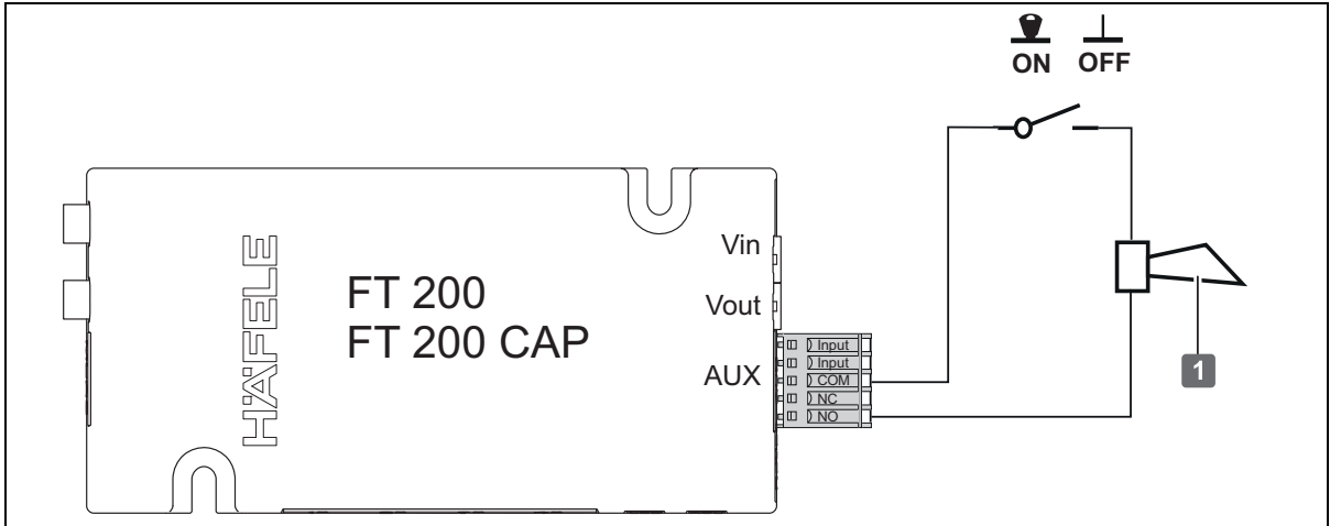
Abb. 5: Installationsbeispiel 2 - FT 200 / FT 200 CAP als Schaltvorrichtung für Alarm [1]
