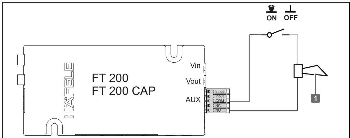
Ilustr. 5: Ejemplo de instalación 2 - FT 200 / FT 200 CAP como dispositivo de conmutación para la alarma [1]
