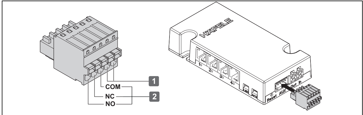
Fig. 3: Collegamenti su ingresso/uscita privo di potenziale
